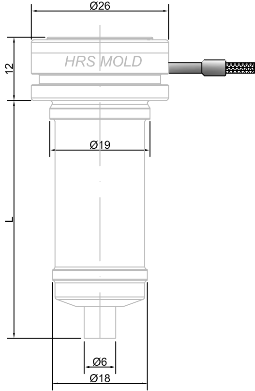
Nozzle Detayı
