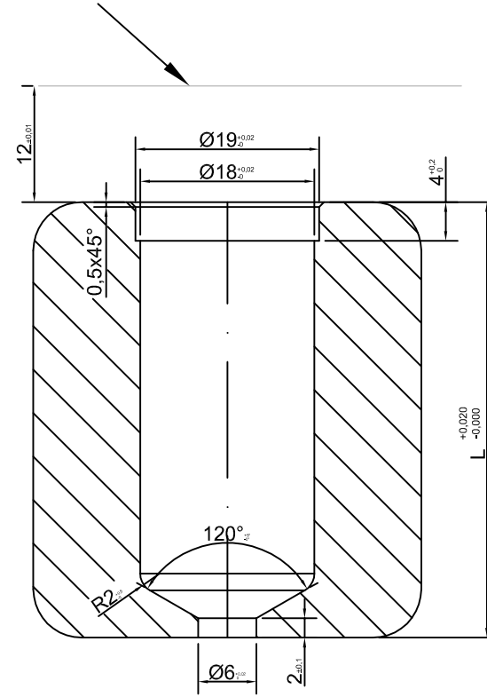
Yuva Detayı
