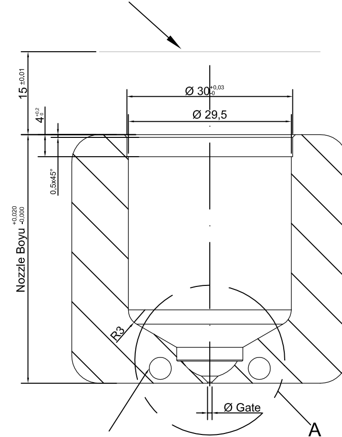
Soğutma Kanalları
