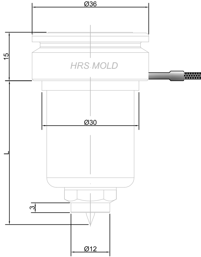
Nozzle Detayı
